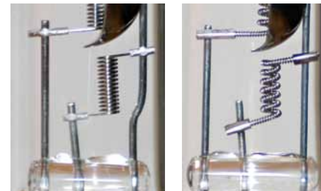
Простая спираль стандартной лампы (слева) по сравнению со стабильной биспиральной нитью оригинальной лампы MAN
